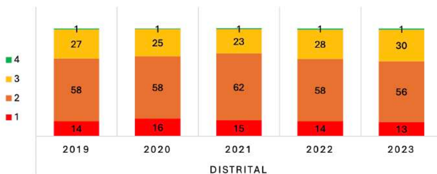
GRÁFICA 4: Saber 11° en la prueba de ciencias naturales 2019 – 2023 Distribución de los estudiantes en los niveles de desempeño
